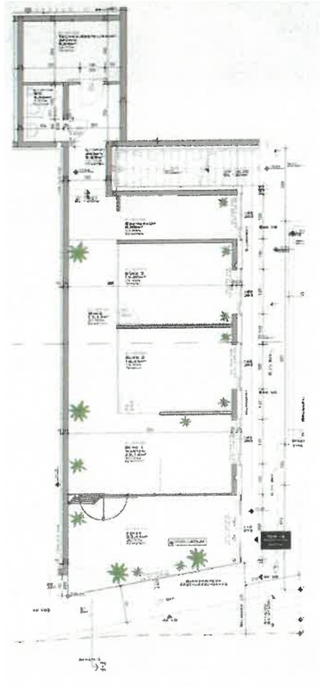
Grundriss
