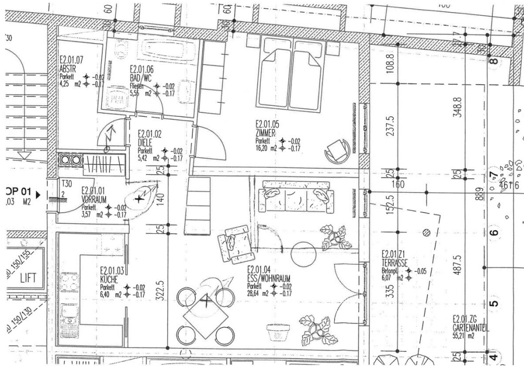
Grundriss
